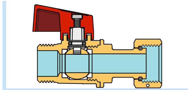
2941 - DETTAGLIO / DETAIL
